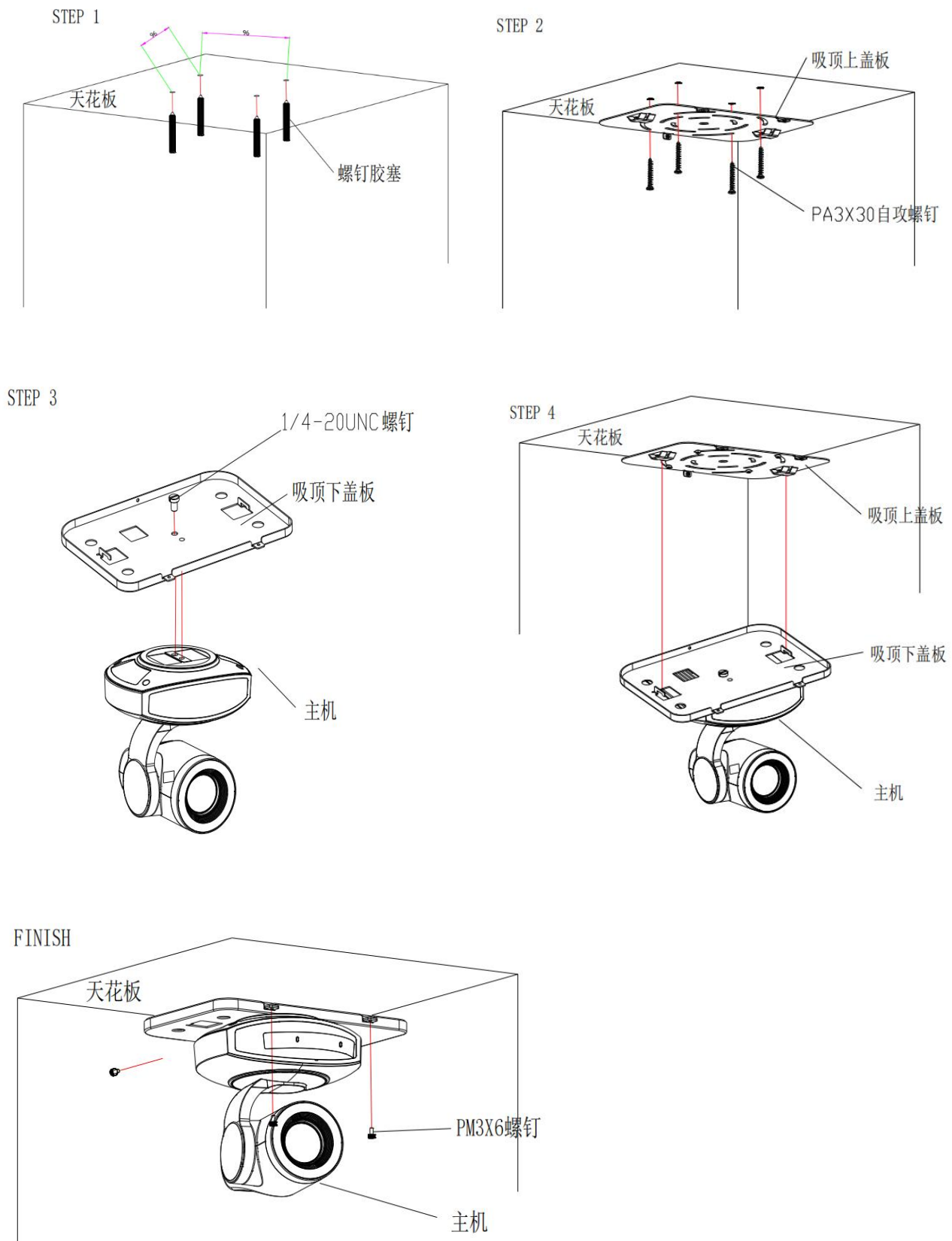
图 1-3 支架倒装步骤
