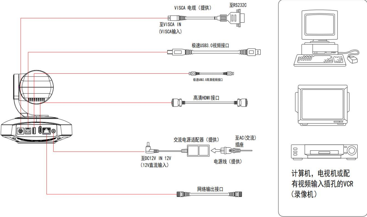
图 2-2 外部接口示意图
