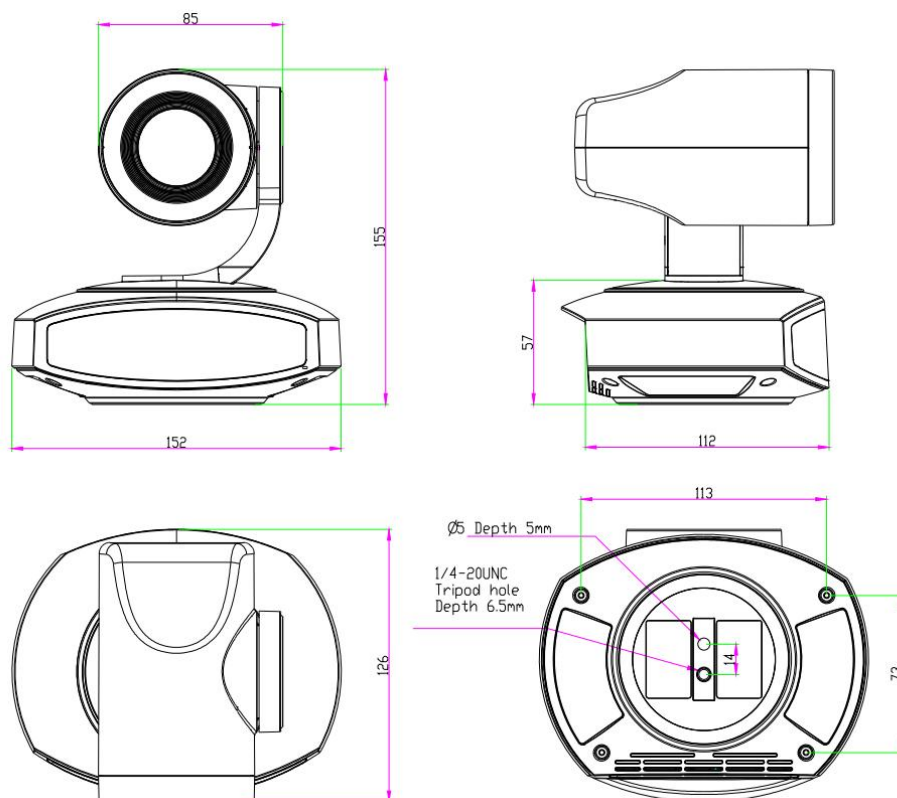
图 2-1 外型尺寸
