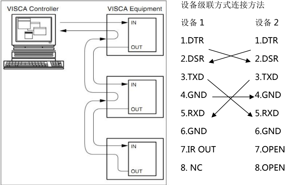
图 2-4 VISCA 组网方式示意图
