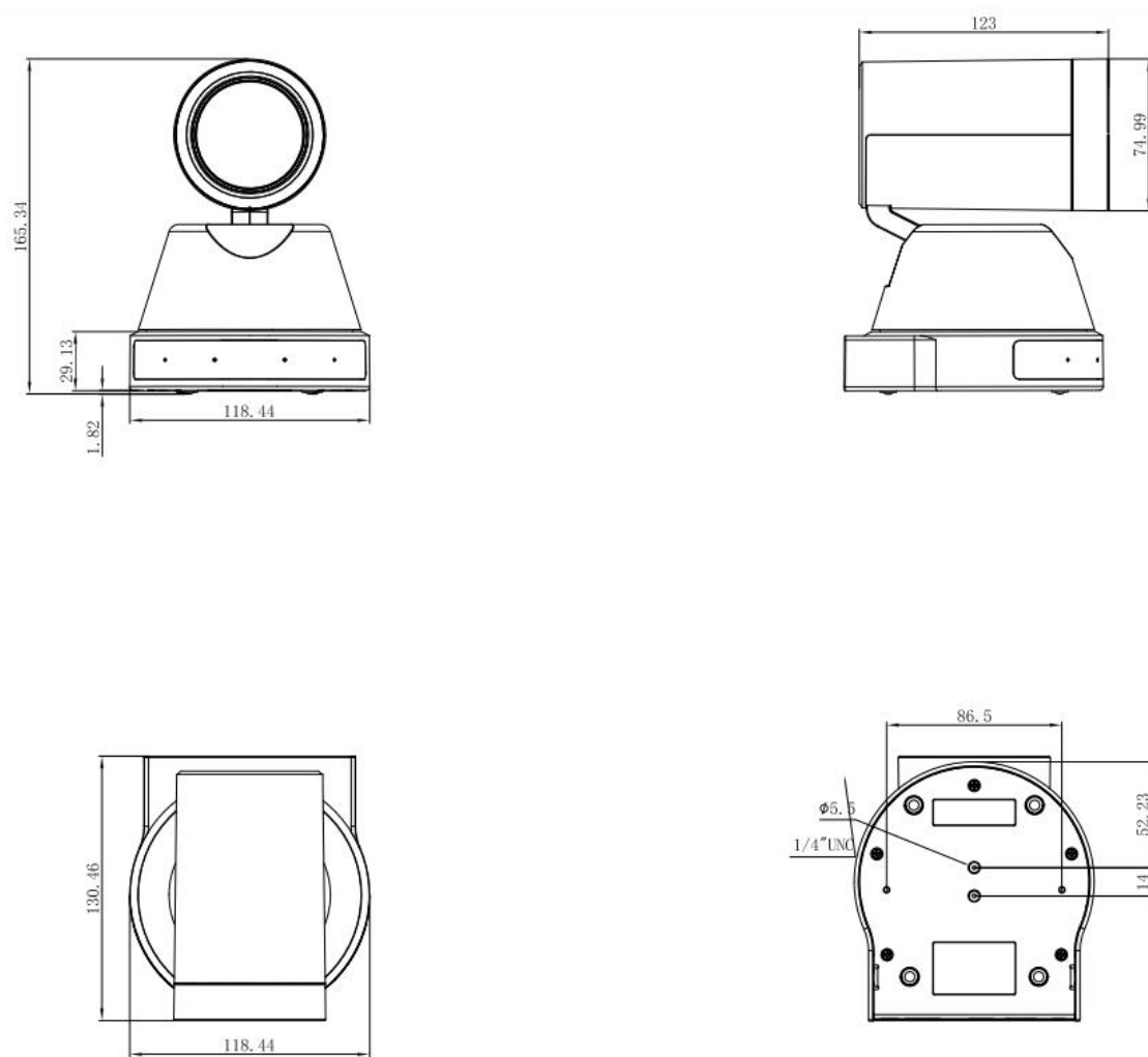
图 2-1 外型尺寸
