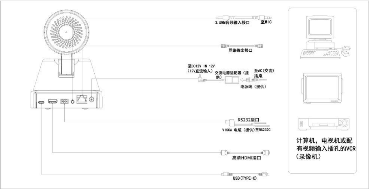
图 2-2 外部接口示意图
