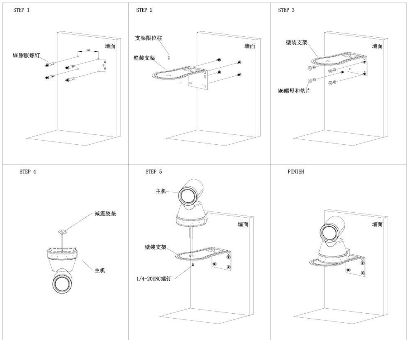
图 1-2 支架正装步骤
