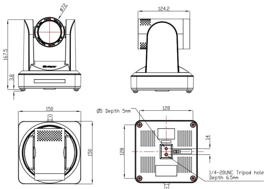
图 2-1 外型尺寸
