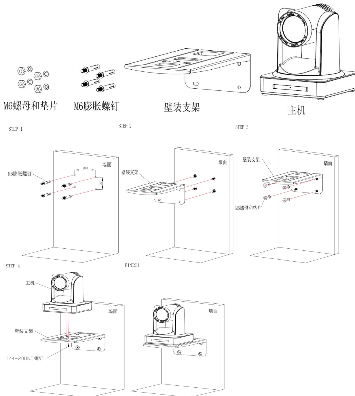
图 1-2 支架正装步骤
