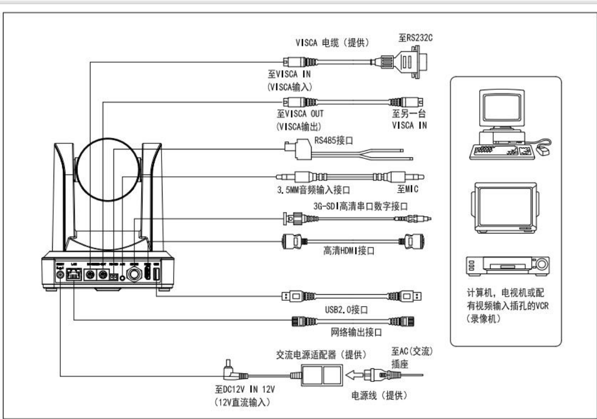
图 2-2 外部接口示意图
