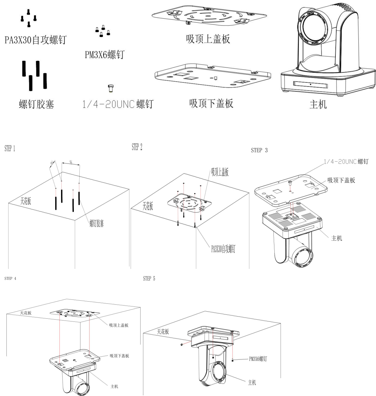
图 1-3 支架倒装步骤
