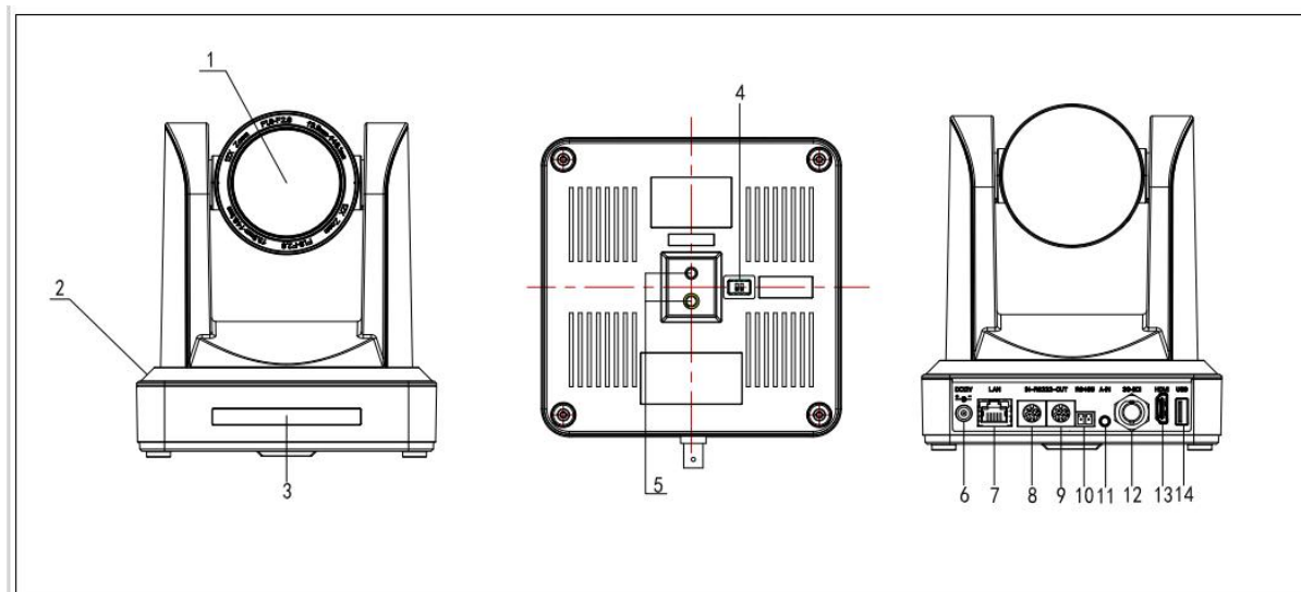
图 1-1 产品接口
